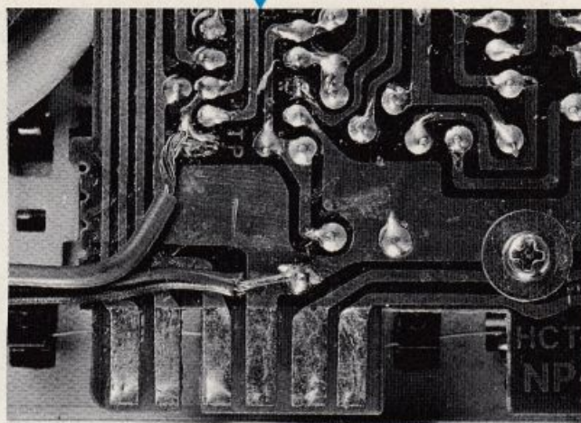
Figura 2. Schema di saldatura dei due fili per il prelievo del segnale di regolazione della testina: al punto TP e alla massa del circuito.
